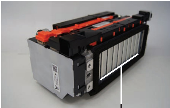
Une des quatre « chaînes » des batteries
