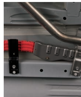
Bouclier thermique près du système d'échappement chaud
